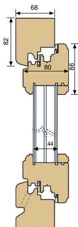
Sezione Verticale Finestra
