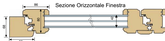
Sezione Orizzontale Finestra
